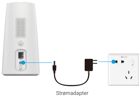
Strømadapter
